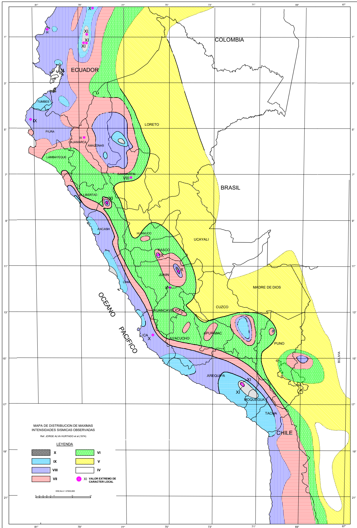
MAPA N° 1 : DISTRIBUCIÓN DE MÁXIMAS INTENSIDADES SÍSMICAS (Alva et al., 1984)
